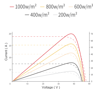
電流-電圧&電力-電圧曲線 (710W)
